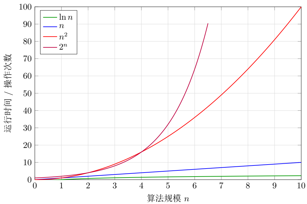
图 1: \ln n 、 n 、 n^2 、 2^n 的增长曲线对比
